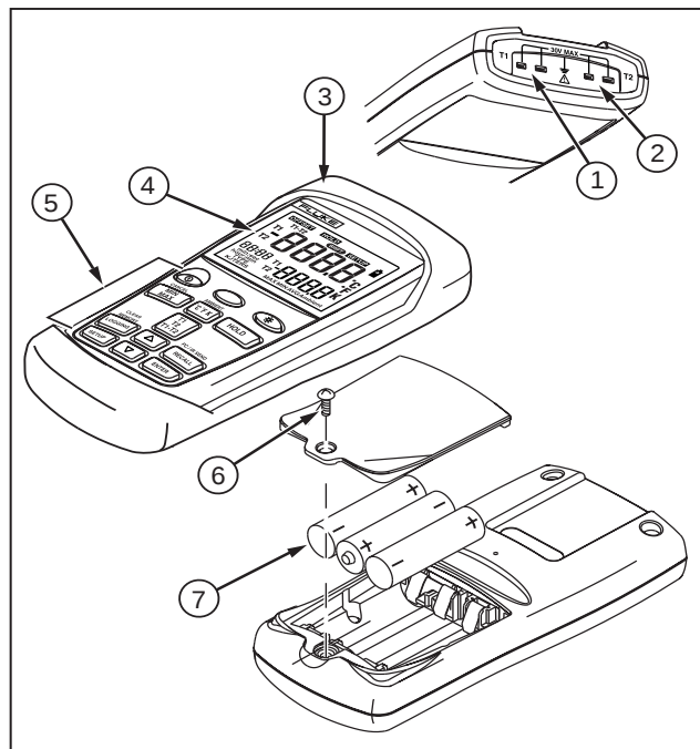
图 1. 部件
