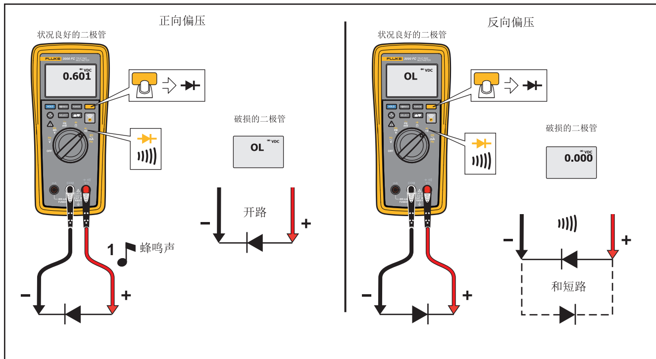
图 7.二极管测试
