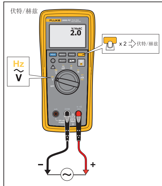
图 2. 伏特/赫兹比
