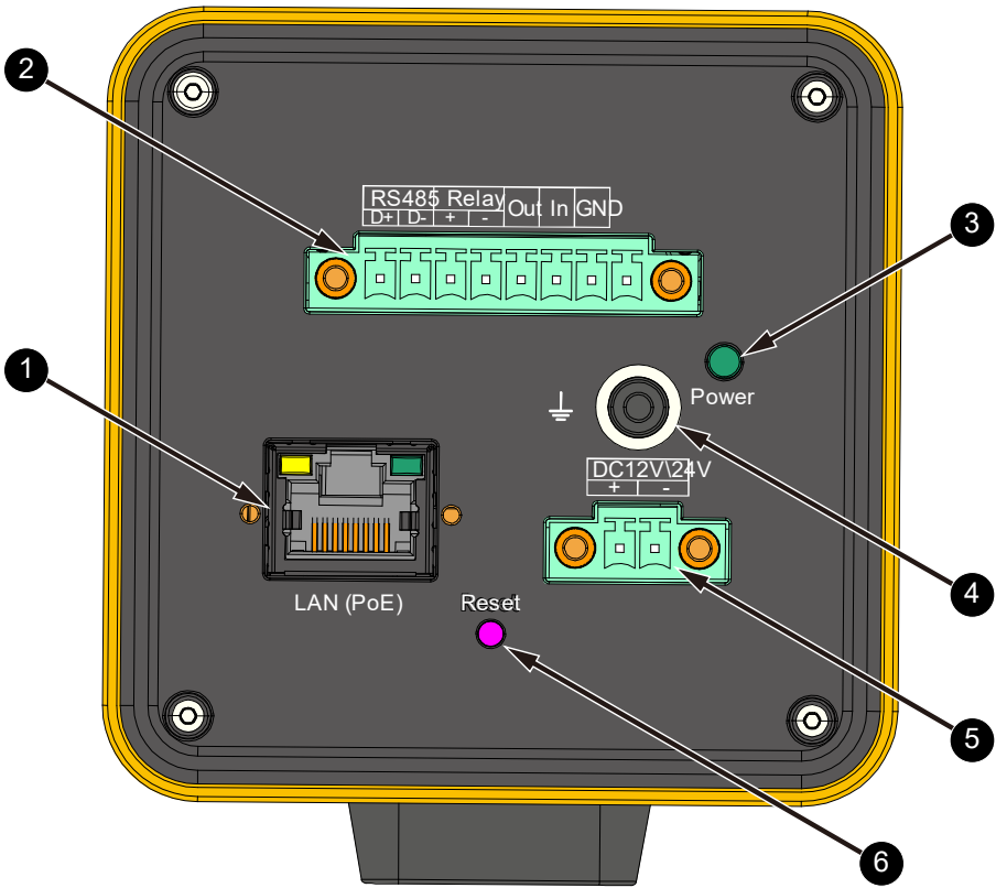
图 5. 产品接口
