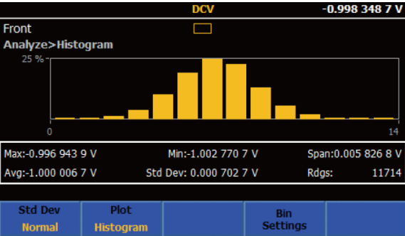
分析：直方图
