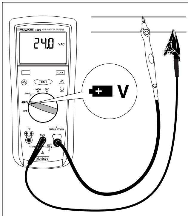
图 5. 测量电压
