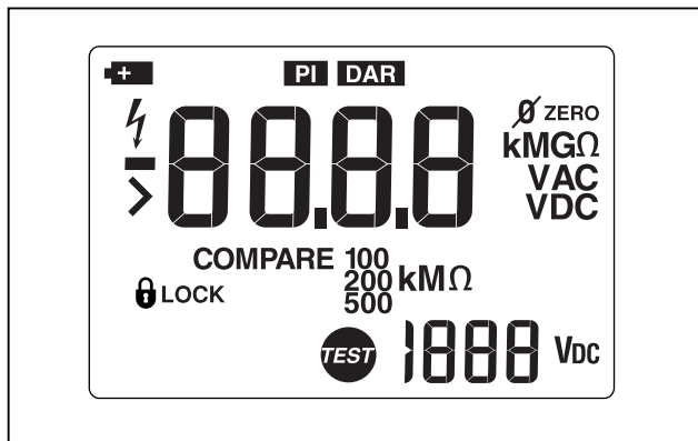
图 3. 显示屏指示符
