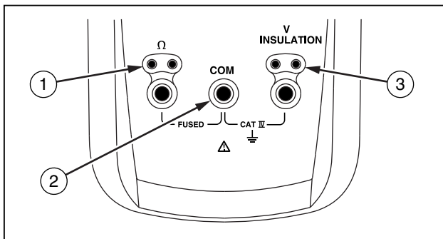
图 4. 输入端子
